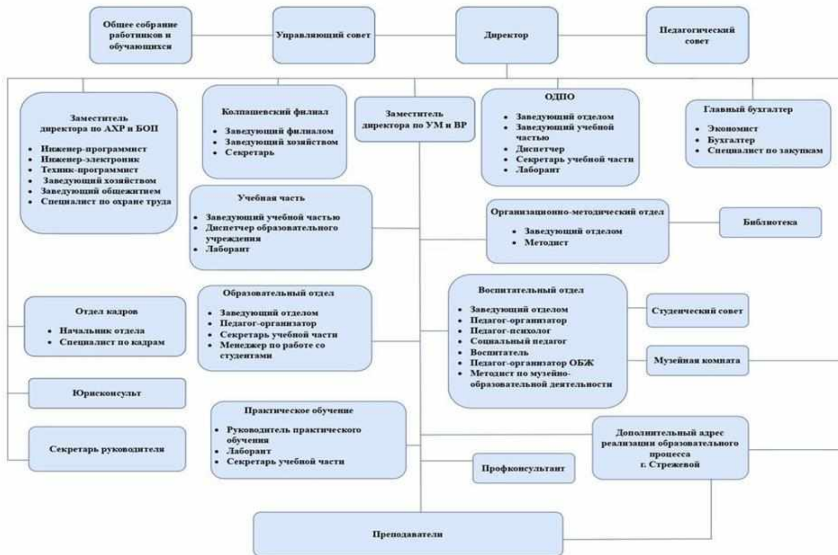
Схема 1. Организационная структура управления Колледже
